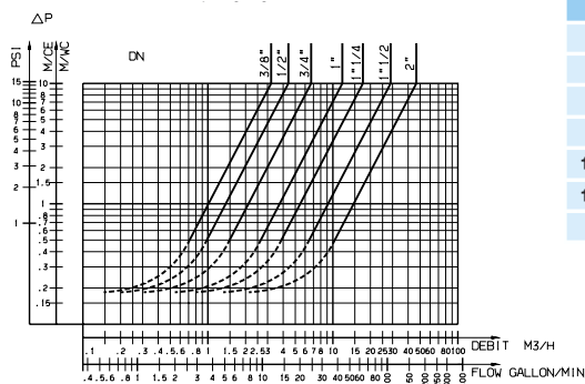
Nyomásveszteségi diagram
