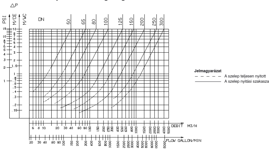
Nyomásvesztési diagram
